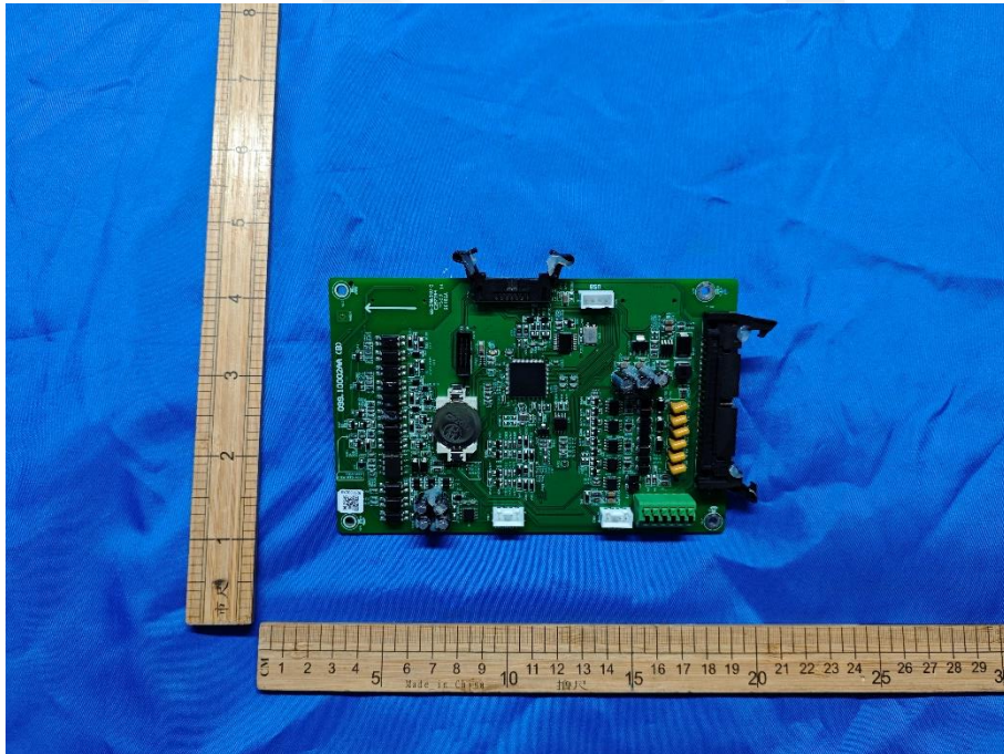
Fig. 14 --PCB view 7
