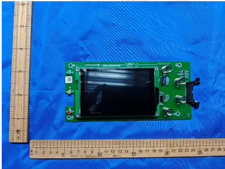
Fig. 16 --PCB view 9
