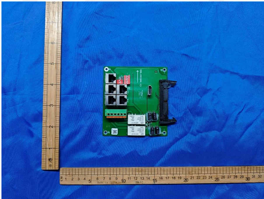
Fig. 12 --PCB view 5
