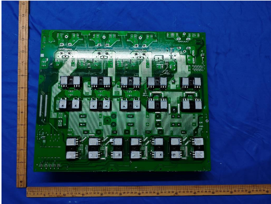
Fig. 11 --PCB view 4
