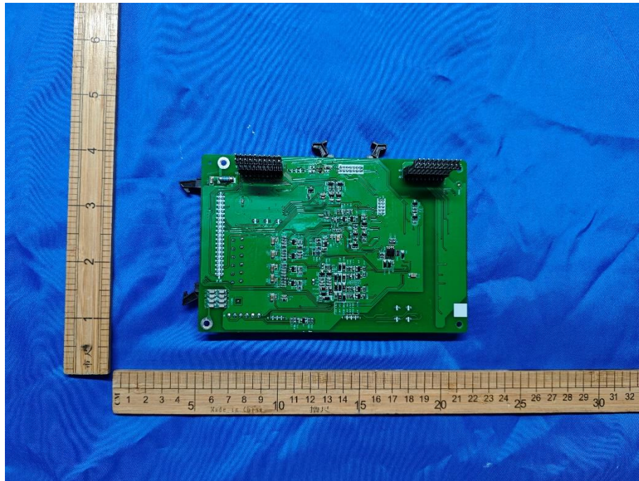
Fig. 15 --PCB view 8
